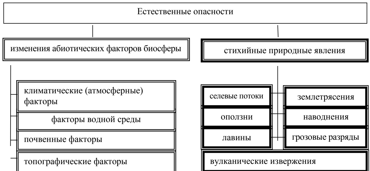
Рисунок 1. Естественные опасности
