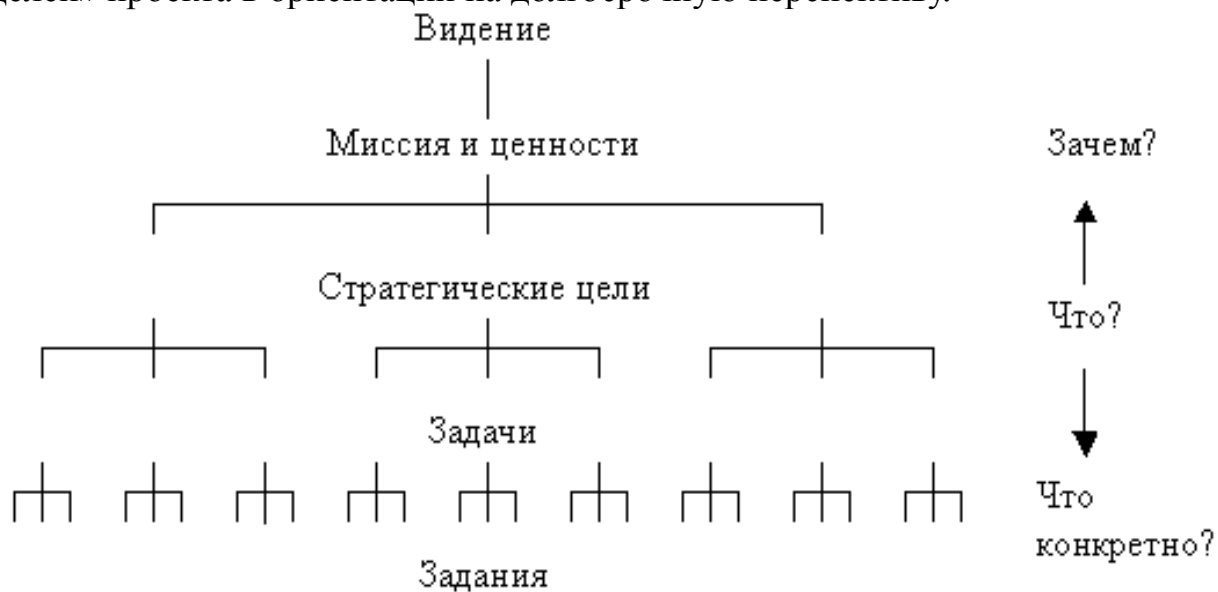
Рис. 1. Дерево целей
